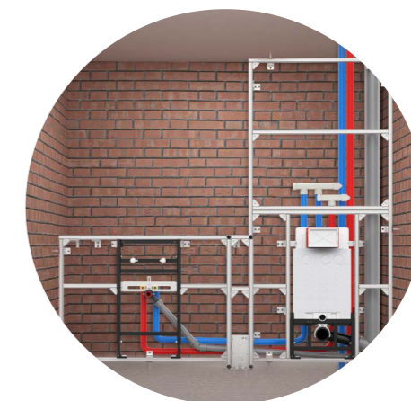
Alcasystem Systémová stěna
